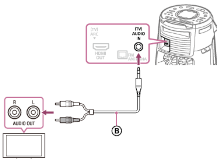
Ⓑ : Аудиокабель (не прилагается)
