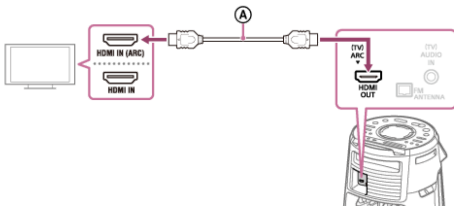
Ⓐ : Высокоскоростной кабель HDMI с Ethernet (не прилагается)
